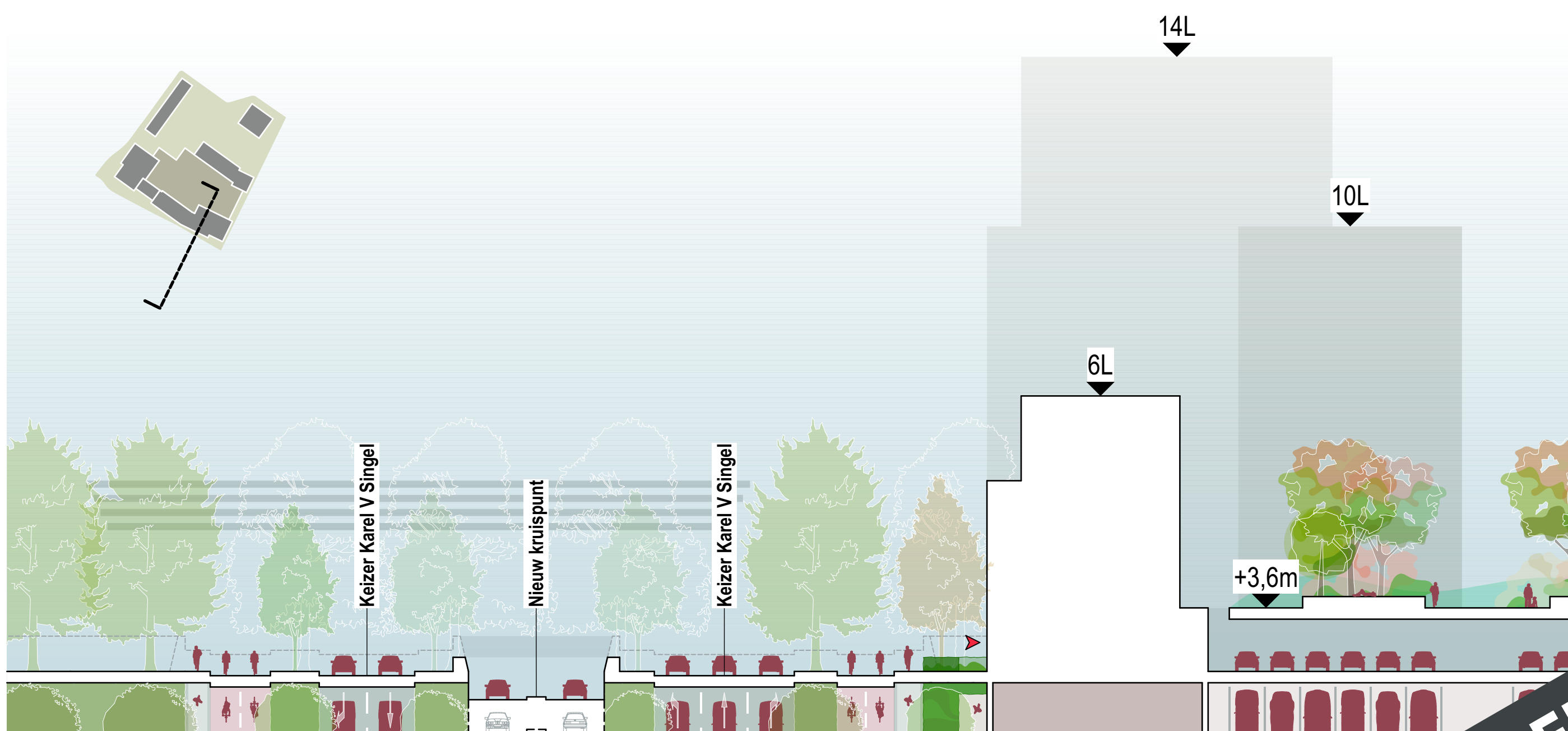
Doorsnede_ Kruispunt en Karel de Grotelaan
