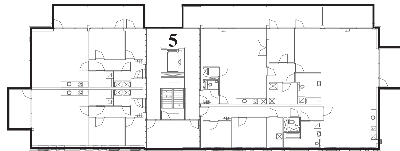
blok 6 en 7 eerste verdieping
